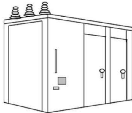
BANCO DE CAPACITORES EN GABINETE CERRADO
